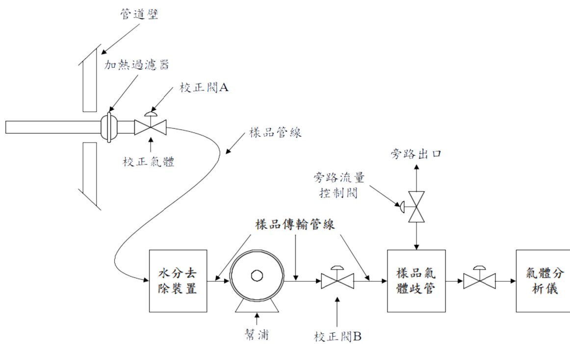
附圖、現場檢測儀器配置示意圖
